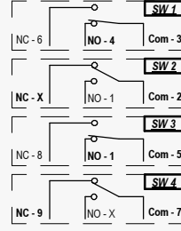
Fırın Kapısı Açık / Oven Door Open, Pyro Kilit Aktif Değil Switch Durum / Pyro Lock Not Active Switch Status
